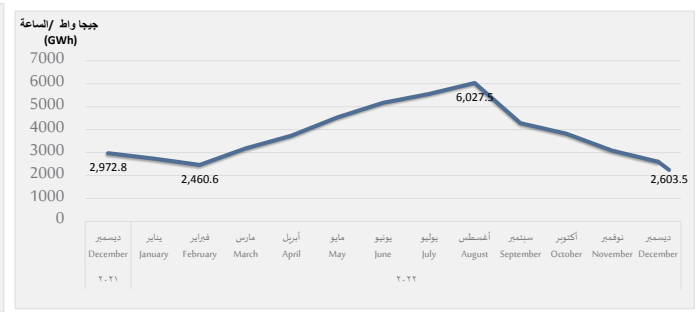
التغير في استخدام الكهرباء، ديسمبر ٢٠٢١ - ديسمبر ٢٠٢٢ Change in Electricity Utilization, Dec. 2021 - Dec. 2022
